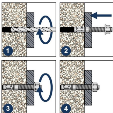
Анкер клиновой с гайкой
