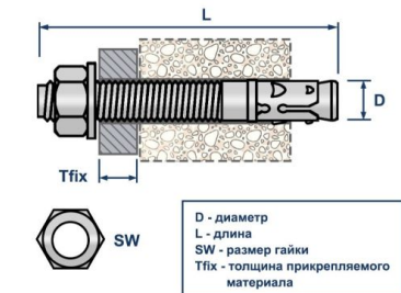
Анкер клиновой с гайкой
