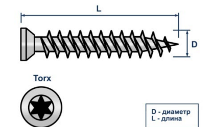
Шуруп нагель по бетону
